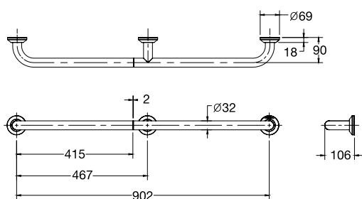
K-45120X-BS ราวจองตัวแบบตรง 90 ซม. Grab Bar 90 cm.
