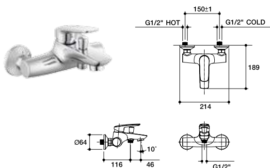
K-76954X-4-CP ก๊อกผสมลงอ่างและยืนอาบแบบก้านโยก ชนิดติดตั้งสำหรับฝักบัวสายอ่อน Aricia Single Lever Exposed Bath and Shower Mixer
