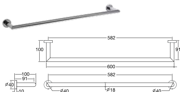
K-13089X-CP ราวแขวนผ้าเดี่ยว 60 ซม. 60 cm. Single Towel Bar
