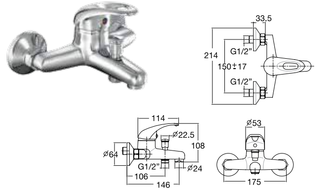
K-15711X-4-CP ก๊อกผสมลงอ่างและยืนอาบแบบก้านโยก ชนิดติดตั้งผนัง สำหรับฝักบัวสายอ่อน Single Lever Exposed Bath and Shower Mixer
