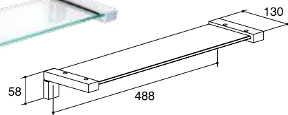
K-72566X-CP ชั้นวางของแบบกระจก/Glass Shelf
