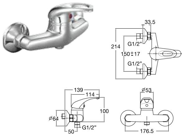
K-15712X-4-CP ก๊อกผสมยืนอาบแบบก้านโยก ชนิดติดตั้งผนัง สำหรับฝักบัวสายอ่อน Single Lever Exposed Shower Mixer
