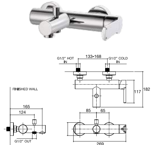
K-98080X-4-CP ก๊อกผสมลงอ่างและยืนอาบแบบก้านโยก ชนิดติดตั้งผนัง สำหรับฝักบัวสายอ่อน Single Lever Exposed Bath and Shower Mixer
