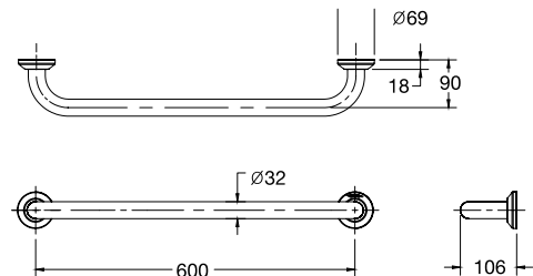
K-45118X-BS ราวจองตัวแบบตรง 60 ซม. Grab Bar 60 cm.
