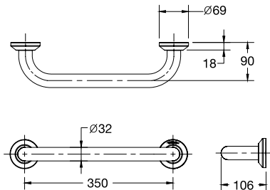
K-45116X-BS ราวจองตัวแบบตรง 35 ซม. Grab Bar 35 cm.
