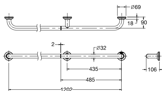
K-45122X-BS ราวจองตัวแบบตรง 120 ซม. Grab Bar 120 cm.
