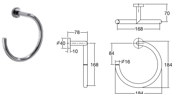
K-13085X-CP ห่วงแขวนผ้าเดี่ยว Towel Ring
