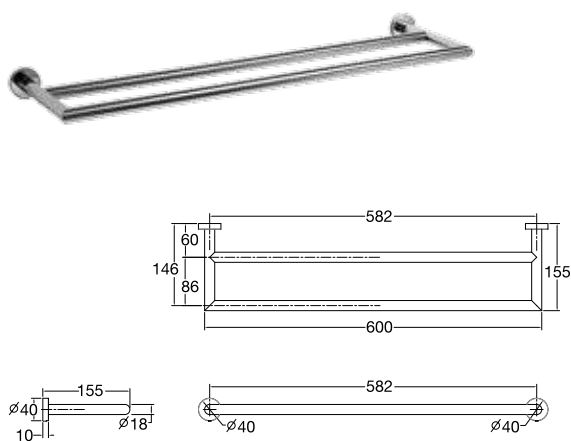
K-13090X-CP ราวแขวนผ้าคู่ 60 ซม. 60 cm. Double Towel Bar
