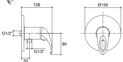
K-15772X-4-CP วาล์วเปิด-ปิดน้ำแบบก้านโยกสำหรับฝักบัวสายอ่อน Single Lever Exposed Shower Valve (Cold Water Only)
