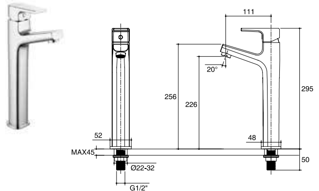
K-98099X-4-CP ก๊อกเดี่ยวอ่างล้างหน้าทรงสูงแบบก้านโยก Single Lever Lavatory Faucet Tall (Cold Water Only)
