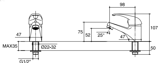
K-15765X-4-CP ก๊อกเดี่ยวอ่างล้างหน้าแบบก้านโยก Single Lever Lavatory Faucet (Cold Water Only)
