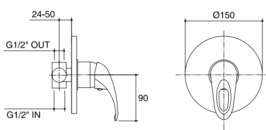
K-16796X-4-CP วาล์วเปิด-ปิดน้ำแบบก้านโยก ชนิดฝังผนังสำหรับฝักบัวก้านแข็ง Single Lever Recessed Shower (Cold Water Only)
