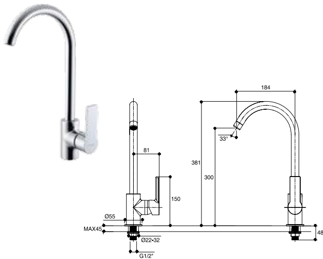
K-98085X-4-CP ก๊อกเดี่ยวอ่างล้างจานแบบก้านโยกชนิดติดตั้งเคาน์เตอร์ Single Lever Kitchen Faucet (Cold Water Only)
