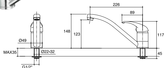
K-15776X-4-CP ก๊อกเดี่ยวอ่างล้างจานแบบก้านโยก Single Lever Kitchen Faucet (Cold Water Only)
