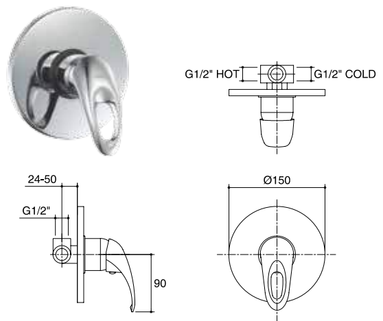
K-15714X-4-CP วาล์วผสมเปิด-ปิดน้ำแบบก้านโยก ชนิดฝังผนัง สำหรับฝักบัวก้านแข็ง Single Lever Recessed Shower Valve Mixer
