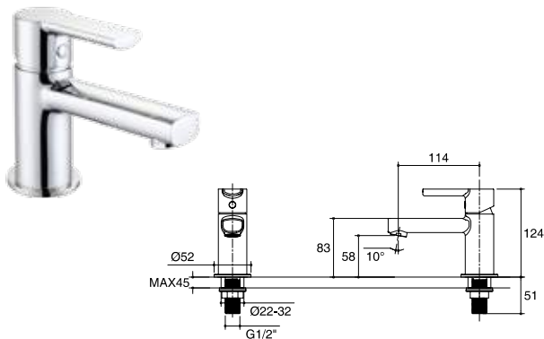
K-98096X-4-CP ก๊อกเดี่ยวอ่างล้างหน้าแบบก้านโยก Single Lever Lavatory Faucet (Cold Water Only)
