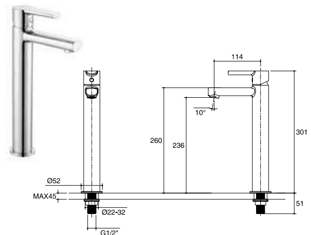
K-98097X-4-CP ก๊อกเดี่ยวอ่างล้างหน้าทรงสูงแบบก้านโยก Single Lever Lavatory Faucet Tall (Cold Water Only)
