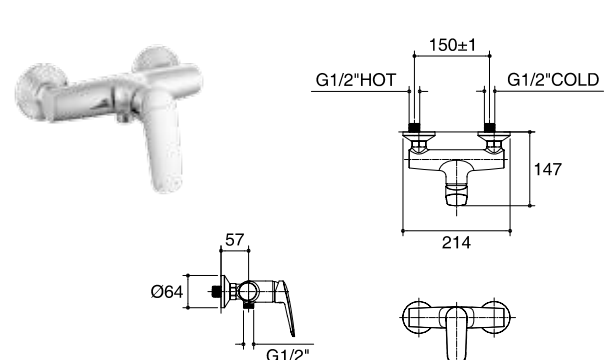
K-76955X-4-CP ก๊อกผสมยืนอาบแบบก้านโยก ชนิดติดตั้งสำหรับฝักบัวสายอ่อน Aricia Single Lever Exposed Shower Valve Mixer
