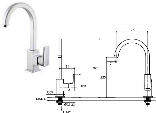
K-98092X-4-CP ก๊อกเดี่ยวอ่างล้างจานแบบก้านโยกชนิดติดเคาน์เตอร์ Single Lever Kitchen Faucet (Cold Water Only)
