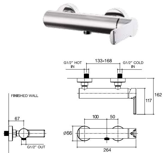
K-98081X-4-CP ก๊อกผสมยืนอาบแบบก้านโยก ชนิดติดตั้งผนัง สำหรับฝักบัวสายอ่อน Single Lever Exposed Shower Mixer
